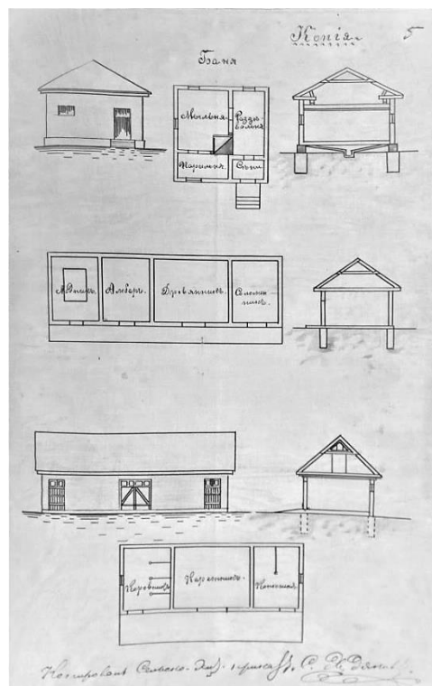
Рисунок 2. Проект/эскиз Приюта для детей Ведомства учреждений Императрицы Марии при починке «Озон» Глазовского уезда Вятской губернии. Фрагмент плана с надворными постройками [9]
