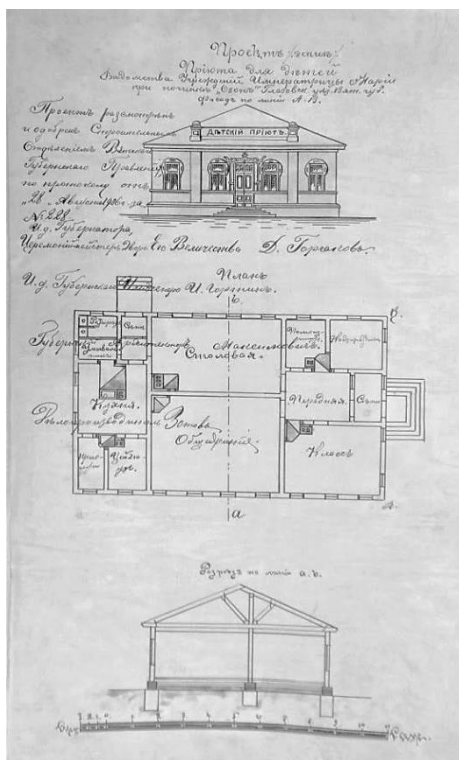
Рисунок 1. Проект/эскиз Приюта для детей Ведомства учреждений Императрицы Марии при починке «Озон» Глазовского уезда Вятской губернии. Фасад и план главного здания [9]
