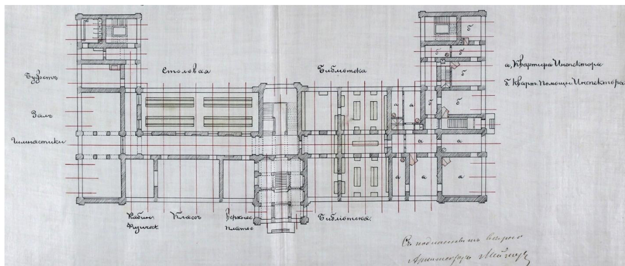
Иллюстрации 1. Фрагмент эскиза Смоленской семинарии. 1 этаж (Государственный архив Смоленской области)
