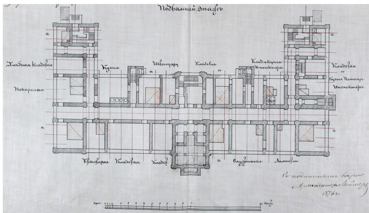
Иллюстрация 4. Фрагмент эскиза Смоленской семинарии. Подвальный этаж (Государственный архив Смоленской области)
