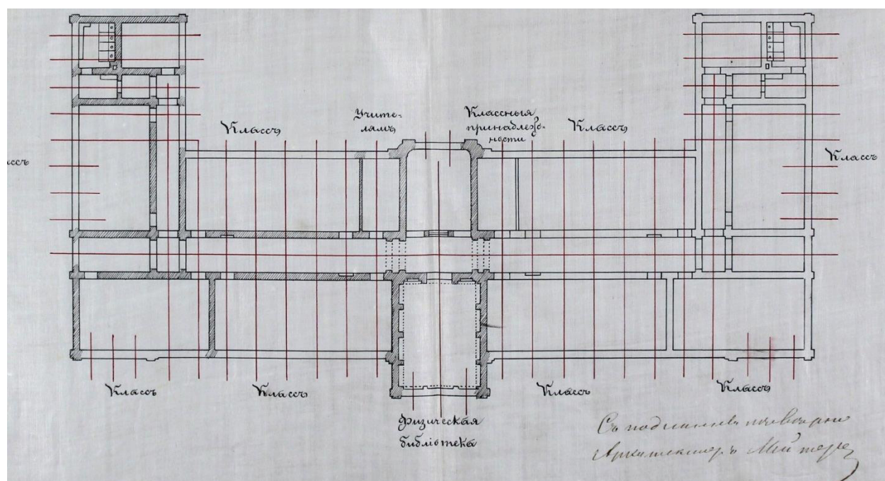
Иллюстрация 2. Фрагмент эскиза Смоленской семинарии. 2 этаж (Государственный архив Смоленской области)
