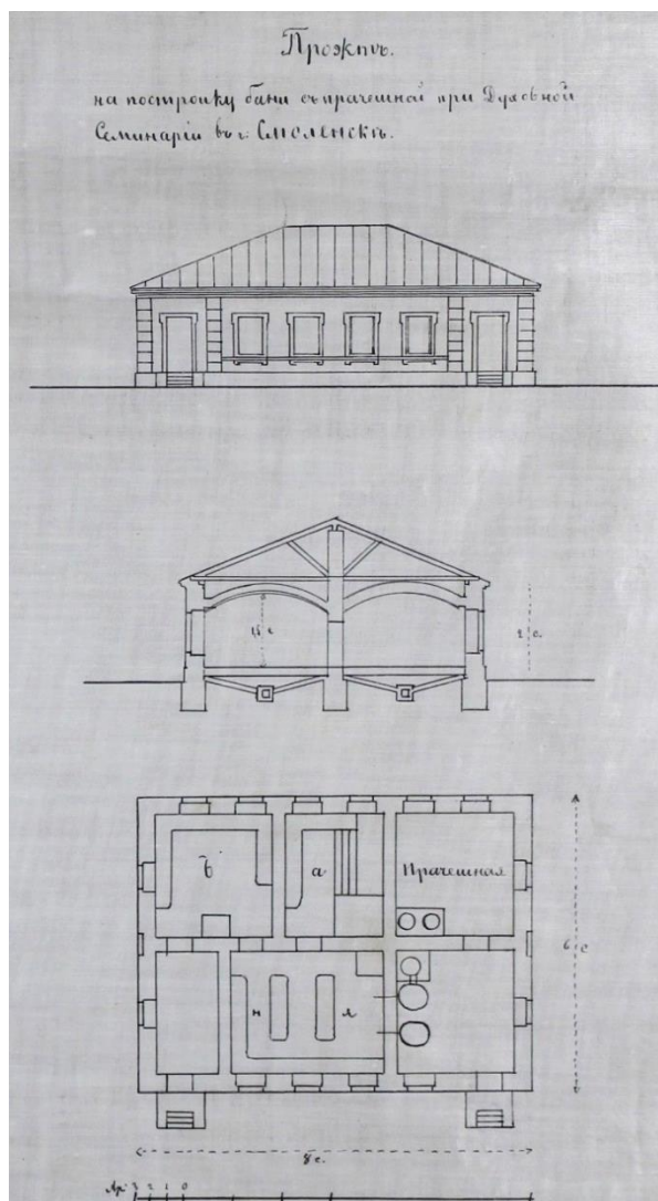
Иллюстрация 5. Фрагмент эскиза Смоленской семинарии. Проект бани и прачечной (Государственный архив Смоленской области)
